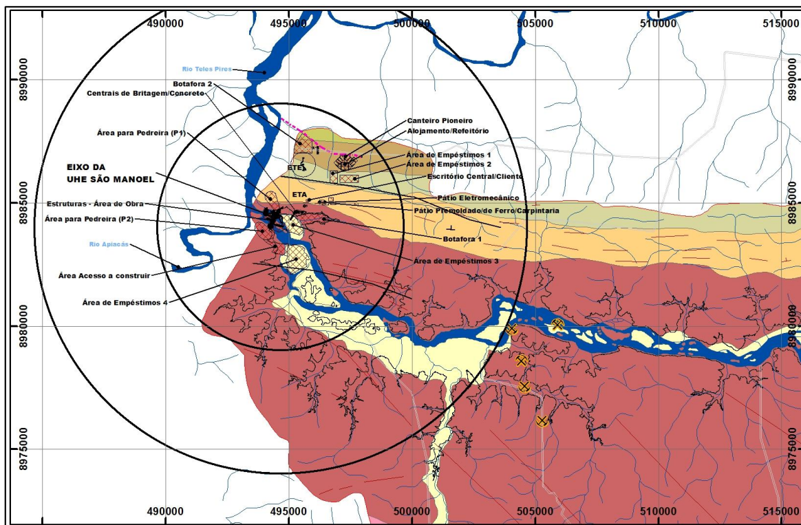
Figura 4 - 2 – Mapa tectônico da porção mais profunda do futuro Reservatório São Manoel.
