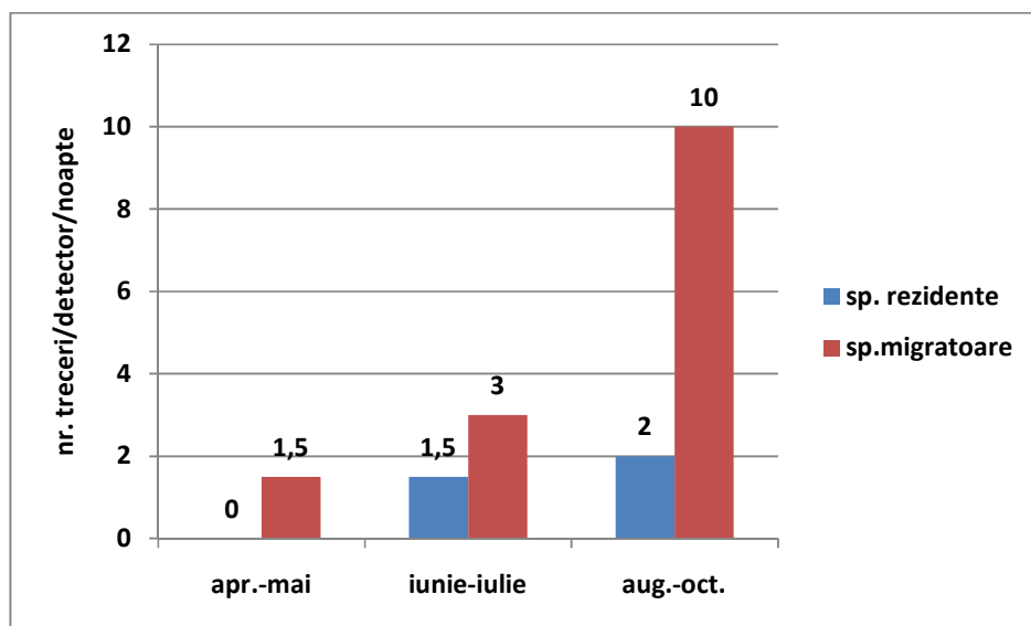
Figura III.9 Numărul total de semnale/detector/noapte înregistrat pentru speciile rezidente și migratoare, în perioada migrației de primăvară (aprilie-mai), în perioada formării coloniilor de naștere (iunie-iulie) și în perioada migrației de toamnă și a împerecherii (august-septembrie)
