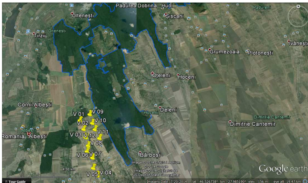
Figura III.3 Punctele de observație din situl Vutcani, linia albastră reprezintă limita ariei protejate ROSCI Pădurea Dobrina-Huși
