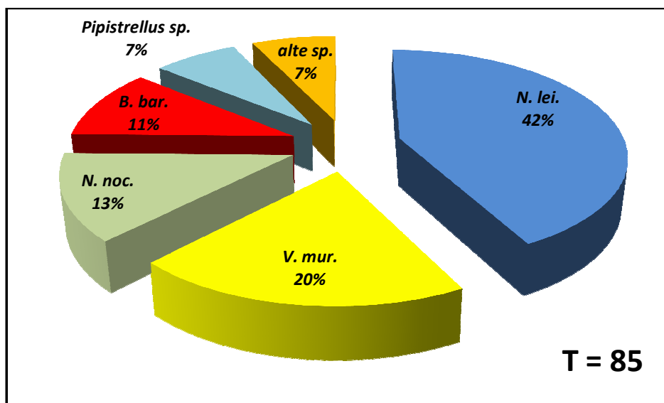
Figura III.4 Abundența speciilor de chiroptere înregistrate în perioada migrației de toamnă și a împerecherii (august-octombrie)
