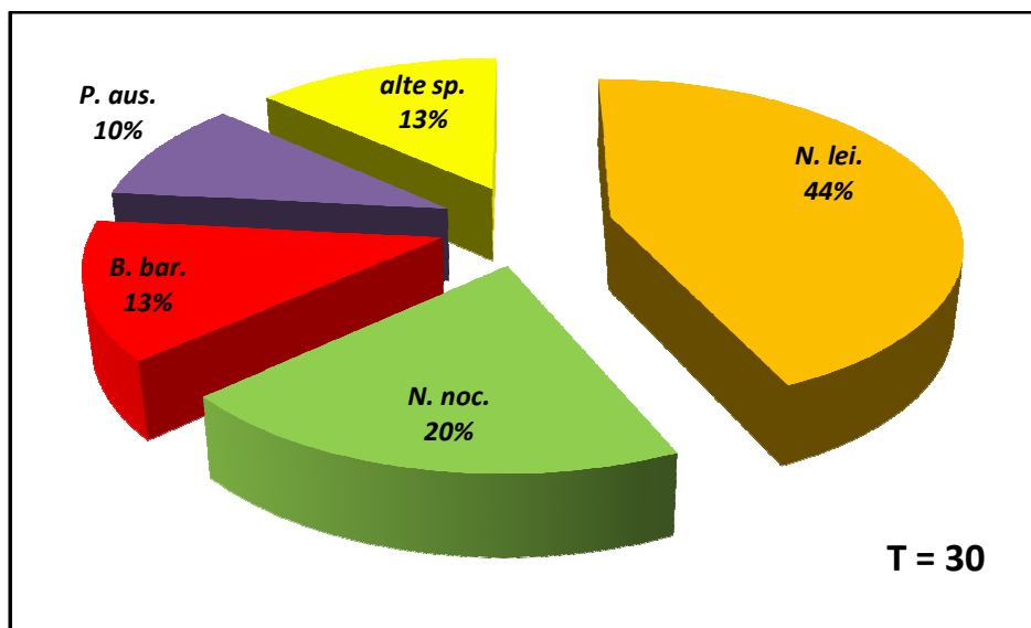
Figura III.6 Abundența speciilor de chiroptere înregistrate în perioada formării coloniilor de naștere (iunie-iulie)
