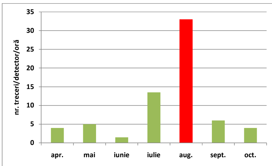
Figura III.8 Numărul total de semnale/detector/oră înregistrat în în lunile calde
