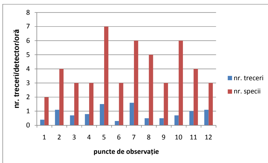
Figura III.10 Numărul total de semnale/detector/oră și numărul de specii identificate în cele 12 puncte, în care au fost efectuate înregistrări în situl Vutcani, în perioada aprilie-octombrie 2013-2014
