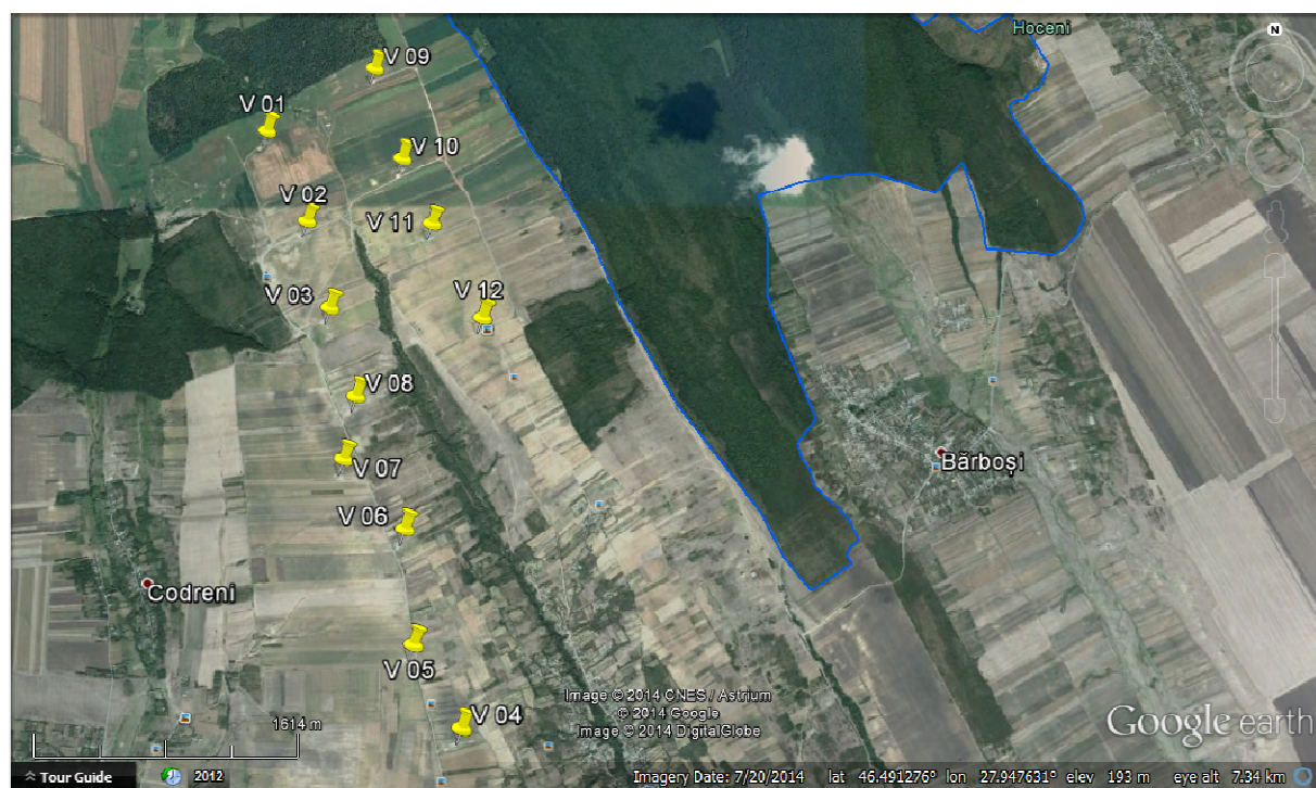
Figura III.2 Punctele de observație din situl Vutcani
