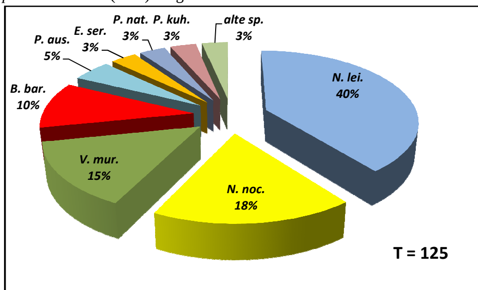
Figura III.1 Compoziția specifică a chiropterelor identificate în parcul de eoliene Vutcani, pe baza detectorului cu expansiune de timp, în perioada septembrie-august 2013-2014. T – reprezintă numărul total de treceri
