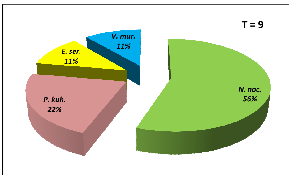
Figura III.5 Abundența speciilor de chiroptere înregistrate în perioada migrației de primăvară (aprilie-mai)
