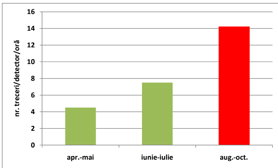
Figura III.7 Numărul total de semnale/detector/oră în perioada migrației de primăvară (aprilie-mai), în perioada formării coloniilor de naștere (iunie-iulie) și în perioada de împerechere și a migrației de toamnă (august-octombrie)
